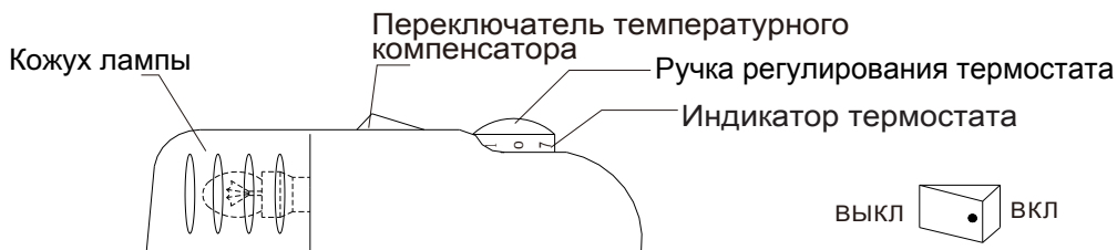
Изображение частей на кожухе термостата
